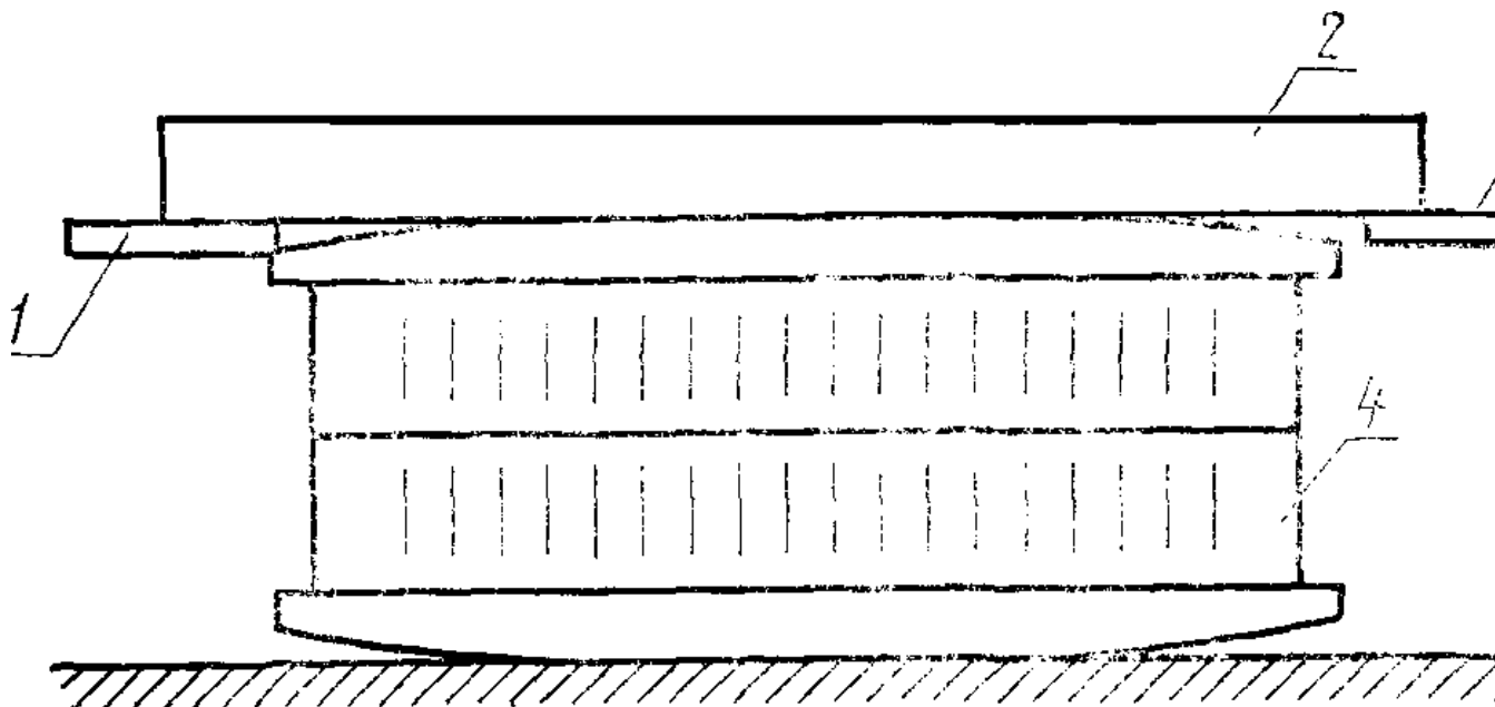
1 - щуп первый; 2 - поверочная линейка; 3 - щуп второй; 4 - блок
