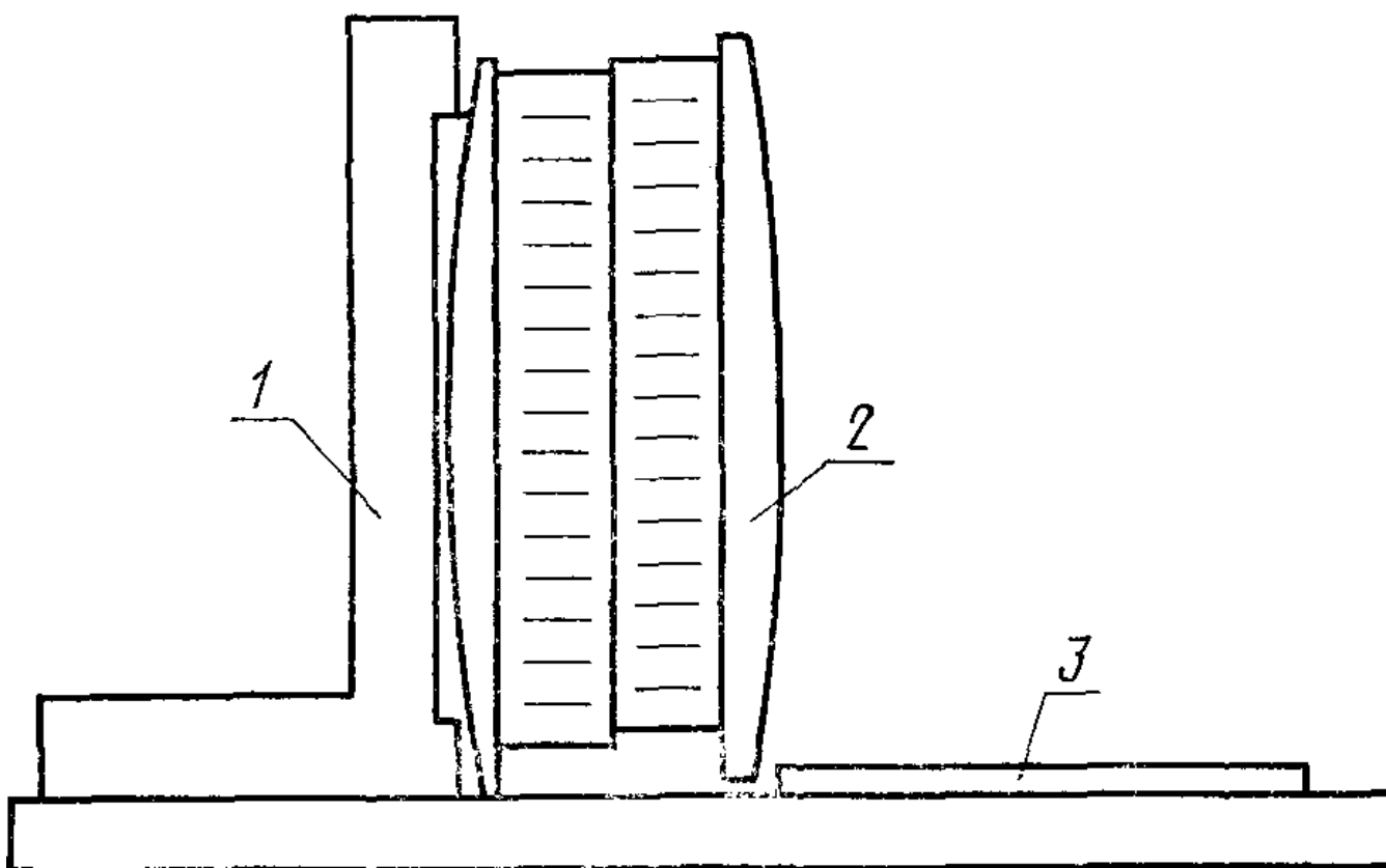
1 - угловая плита; 2 - блок; 3 - щуп; 4 - поперочная плита
