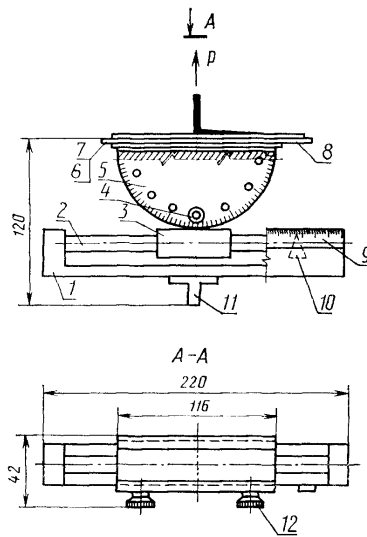
1 - основание; 2 - направляющая; 3 - салазки; 4 - фиксатор; 5 - угломер; 6, 7 - прижимные гайки, планки и винты; 8 - образец; 9 - линейка; 10 - стрелка; 11 - переход; 12 - затяжные гайки Черт. 3
