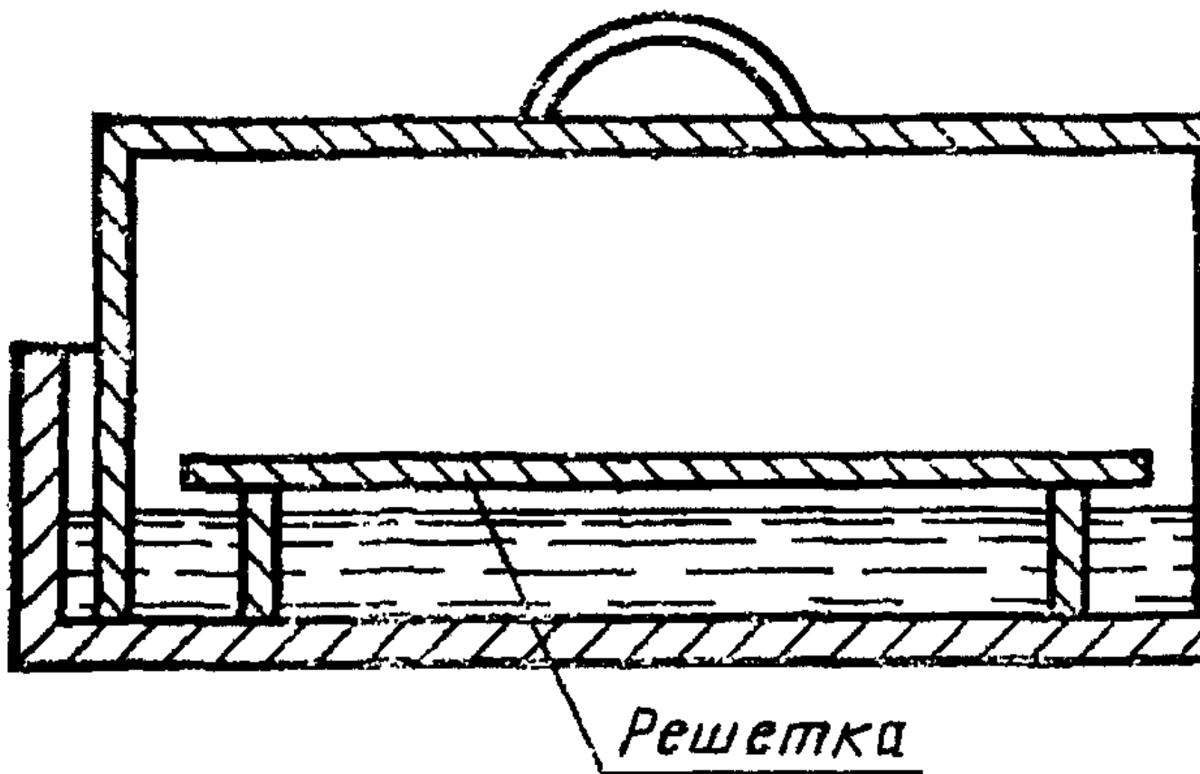
Ванна с гидравлическим затвором
