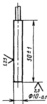
Черт. 2 Рабочая часть пестика
