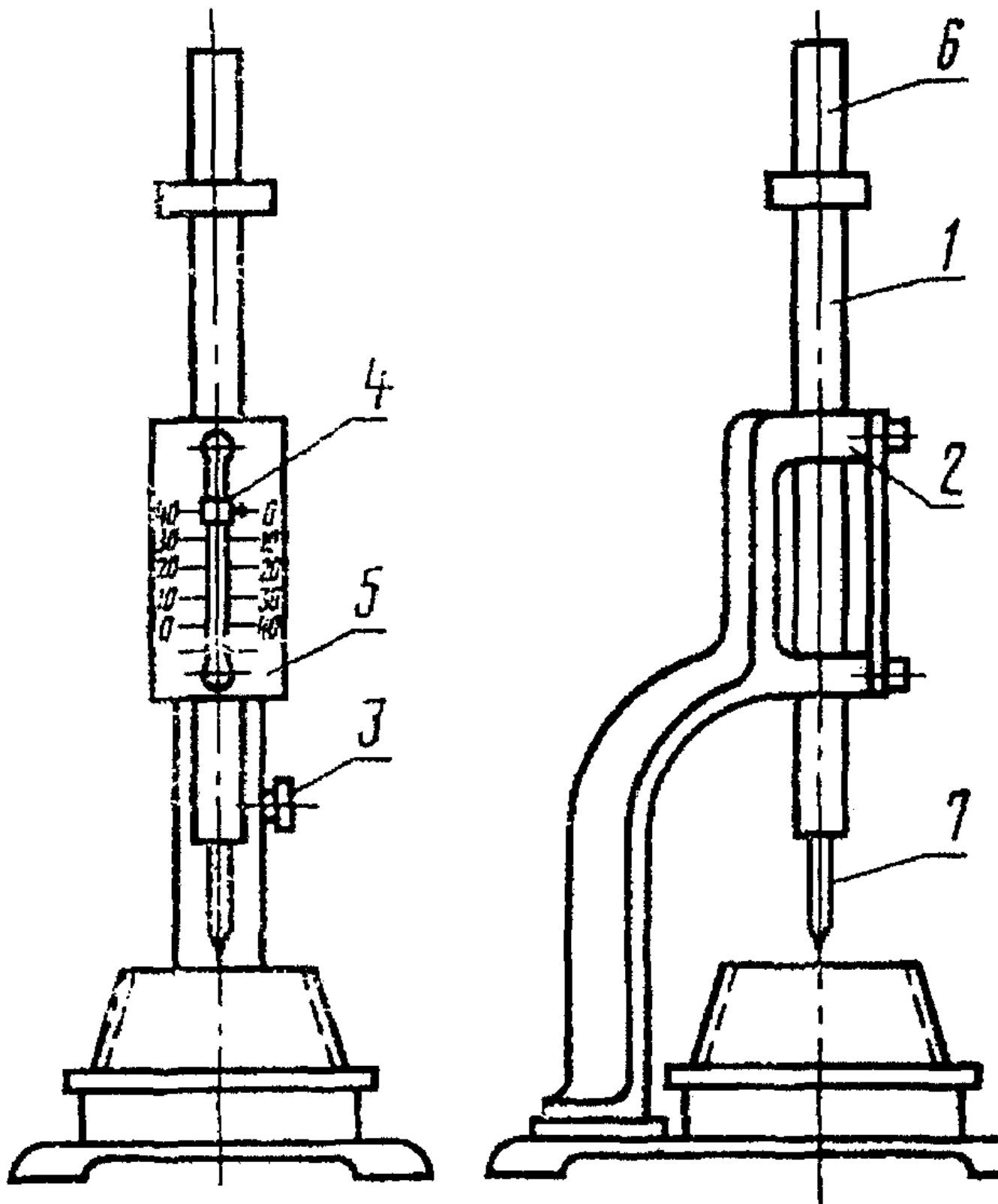
1 - цилиндрический металлический стержень; 2 - обойма станины; 3 - стопорное устройство; 4 - указатель; 5 - шкала; 6 - пестик; 7 - игла
