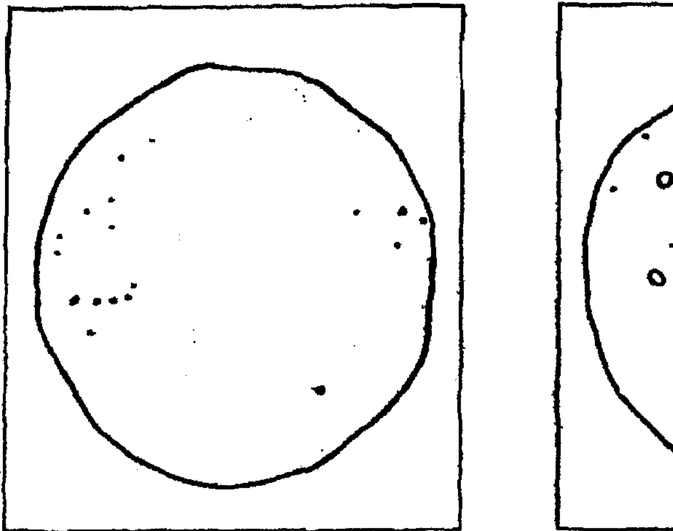
Лепешки, не выдержавшие испытания на равномерность изменения объема
