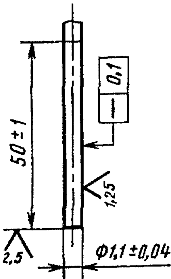
Рабочая часть иглы
