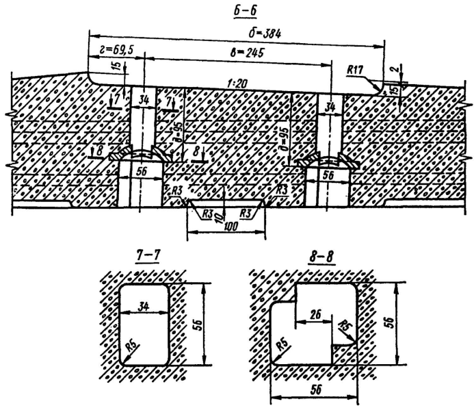
А - вариант очертания поверхности шпалы; Б - арматура показана пунктиром. Черт. 2.
