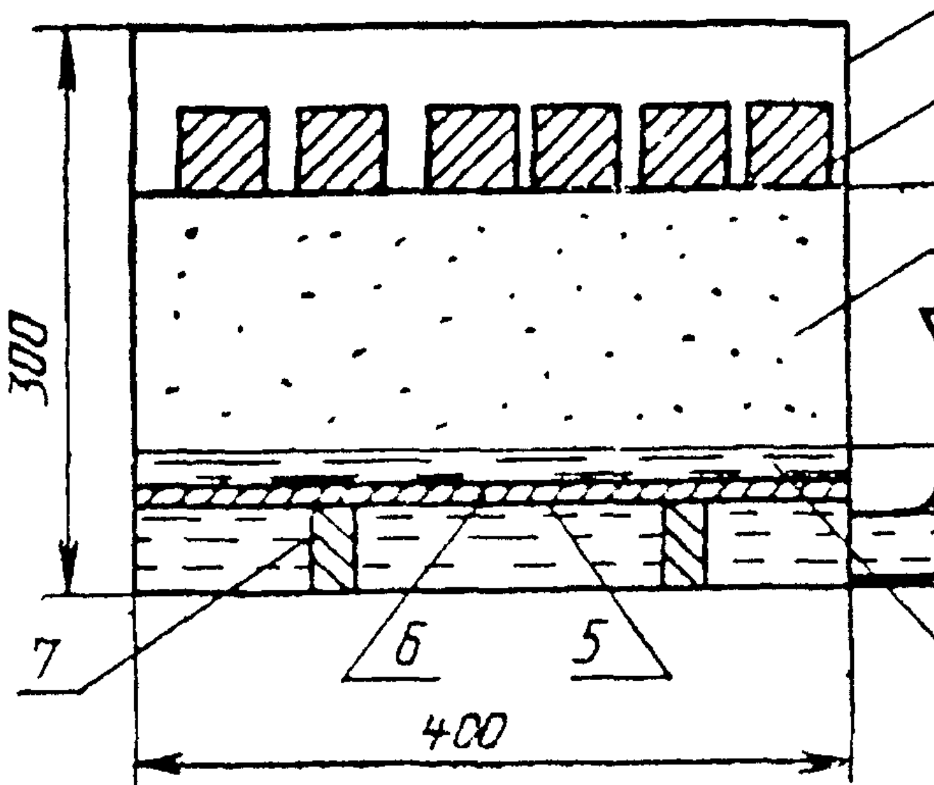
Рисунок 1. Схема устройства для капиллярного водонасыщения образцов
